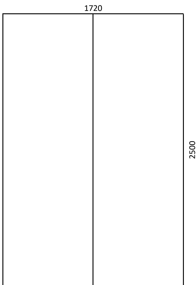
Okno 2 kwaterowe ze słupkiem ruchomym
