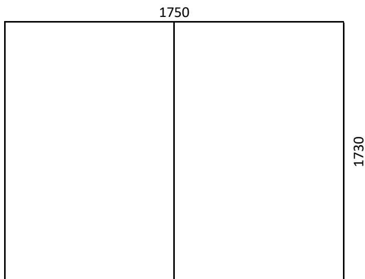
Okno 2 kwaterowe ze słupkiem stałym
